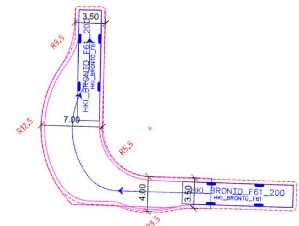
Kuva 1. Nostolavayksikön ajouramalli.
